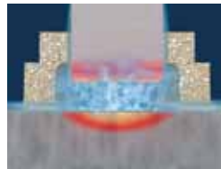
Der Lichtbogen schmilzt Bolzen und Werkstück an.
